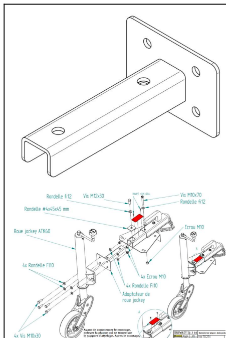
Support central de roue jockey, fourni complet avec nécessaire de montage. S'adapte sur les remorques avec Timon SG950 et 1300 sans frein-Réf K10.213
